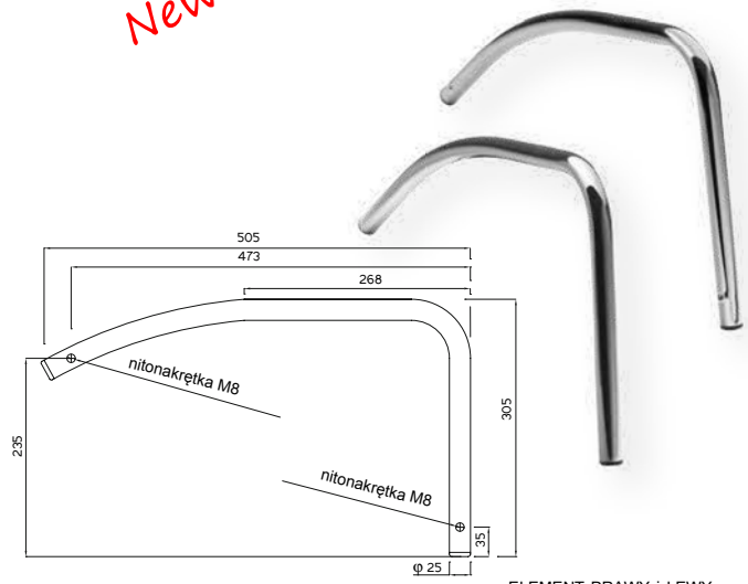
ELEMENT PRAWY I LEWY
