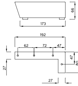
Noga prawa i lewa
