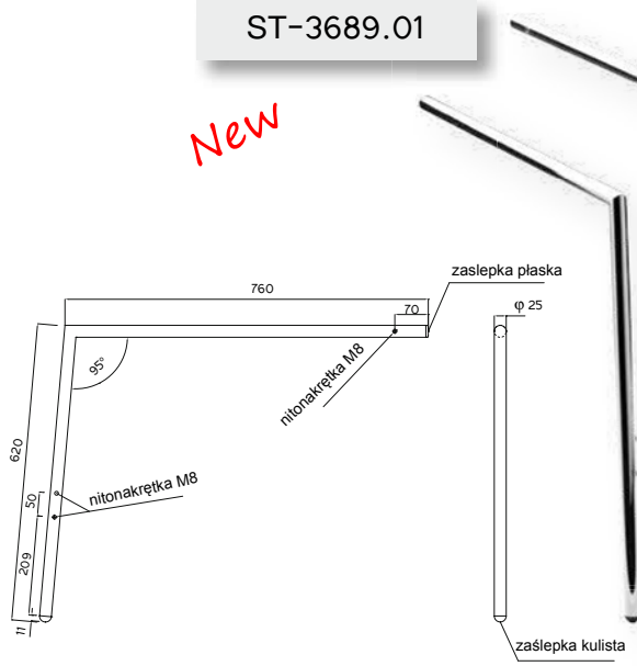
ELEMENT PRAWY I LEWY
